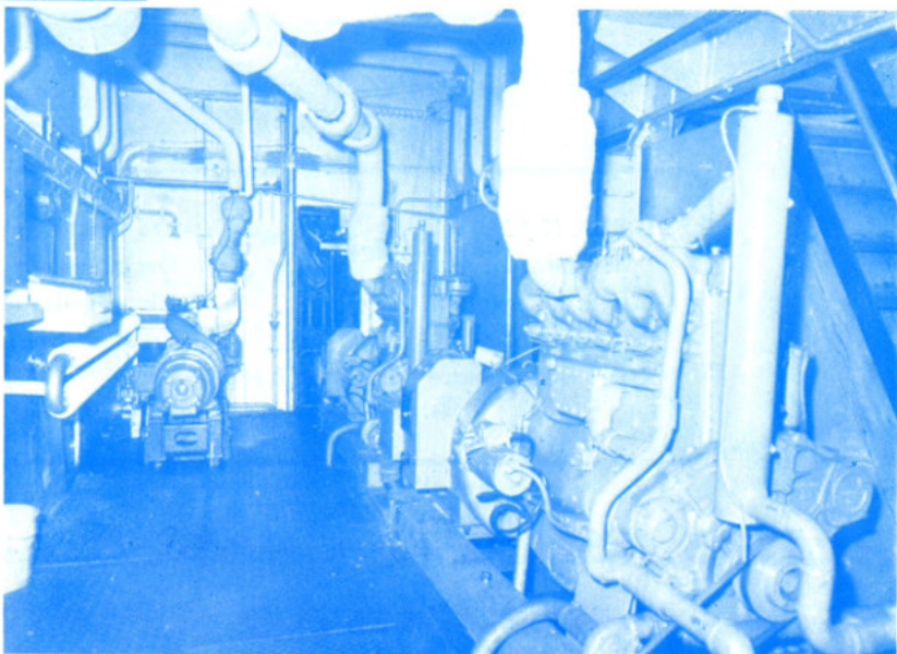
Sändarrum med 2 st. 10.000 Watts sändare av märket Continental.
